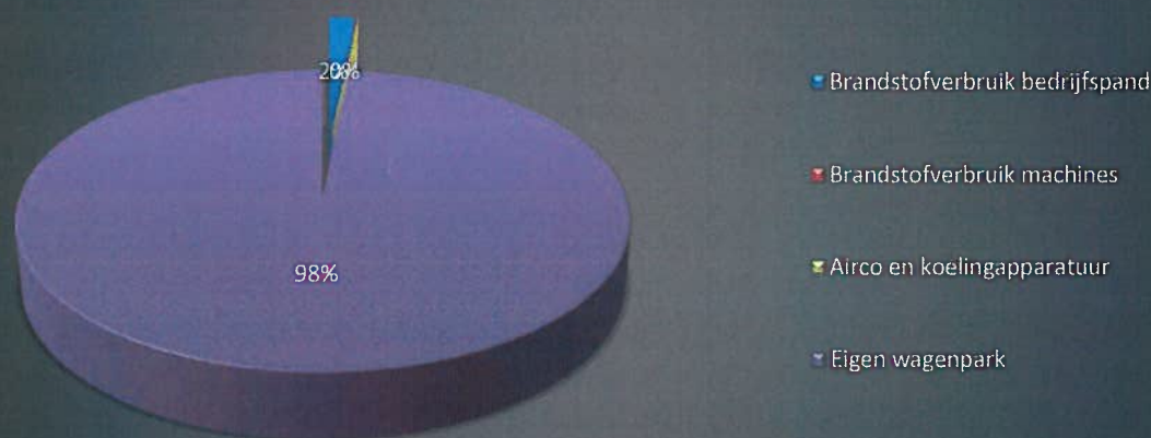
Onderlinge verhoudingen CO 2 -emissie scope 1 - 2013
