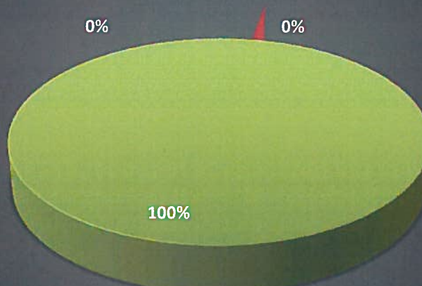
Onderlinge verhoudingen CO 2 -emissie scope 2 - 2014
