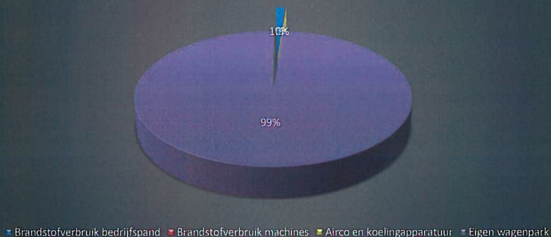
Onderlinge verhoudingen CO 2 -emissie scope 1 - 2014
